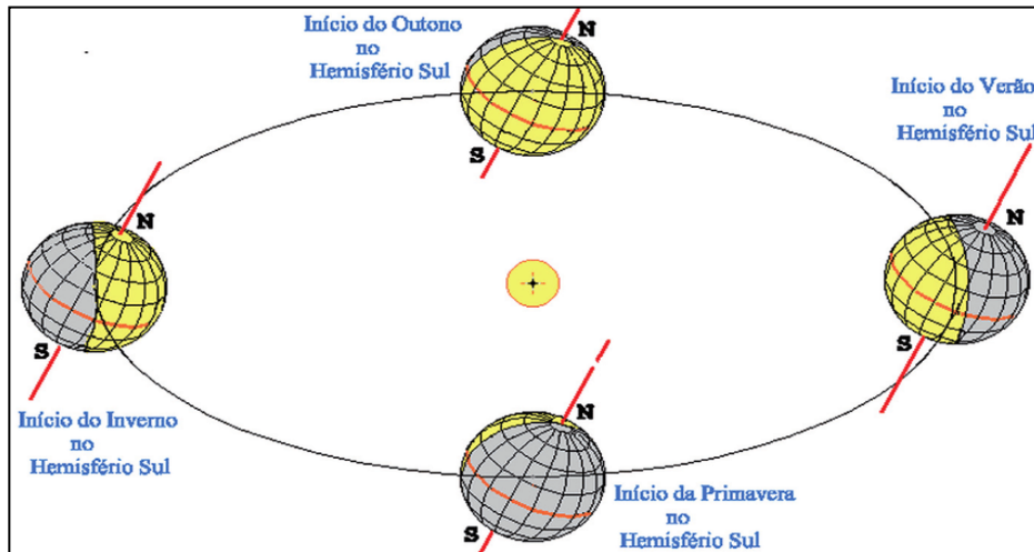
Figura 2: Desenho esquemático representando o início das estações do ano para o hemisfério Sul em quatro posições da órbita da Terra.
